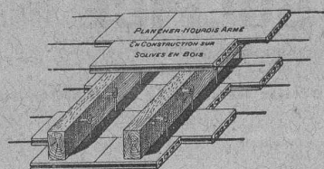
Plafond-hourdis armé s/solives en bois.
