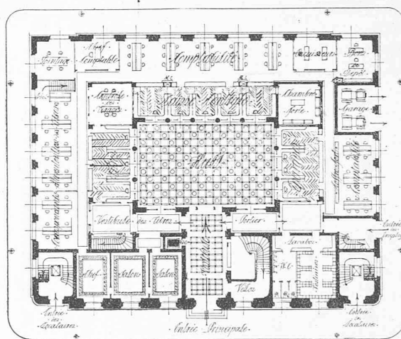
Plan du rez-de-chaussée — 1 : 600.
