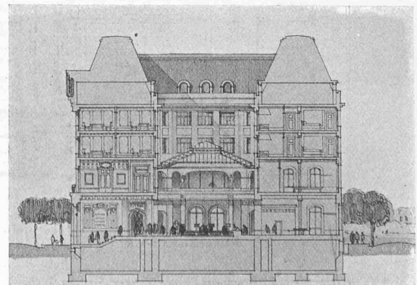
Coupe transversale — 1 : 600
