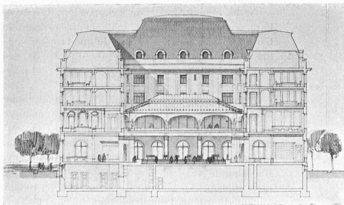
Coupe longitudinale — 1 : 600
