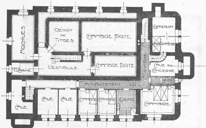
Plan du sous-sol. — 1 : 300.
