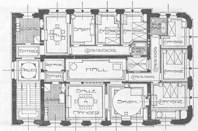
Plan du 2 me étage. — 1 : 300.
