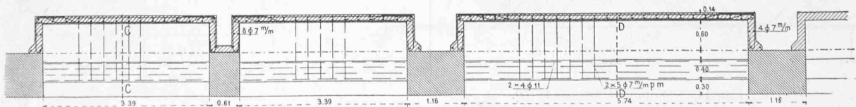
Fig. 23. — Armatures des sauts de loup. — Plan. — 1 : 100.
