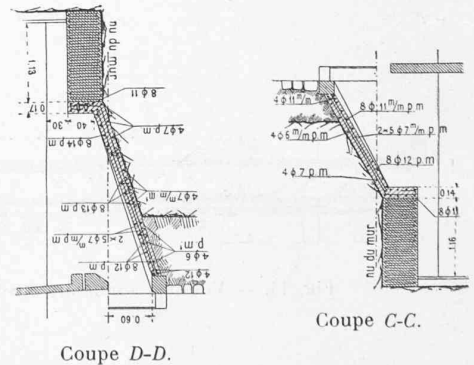
Fig. 24. — Sauts de loup. — 1 : 100.
