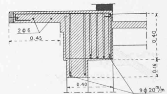
Fig. 15. — Couvertes 820-821. — 1 : 30.
