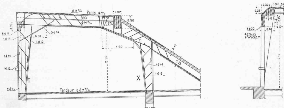
Fig. 19. — Vue du sommier 903 et des piliers I-X. — 1 : 80.
