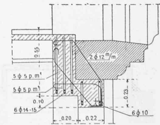
Fig. 16. — Couverte 802. — 1 : 30.
