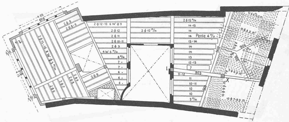
Fig. 17. — Toiture en béton armé. — 1 : 200.
