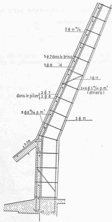
Fig. 7. — Armature du brisis au 4 e étage. — 1 : 30.
