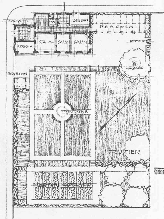
Villa D. - 1 : 300.
