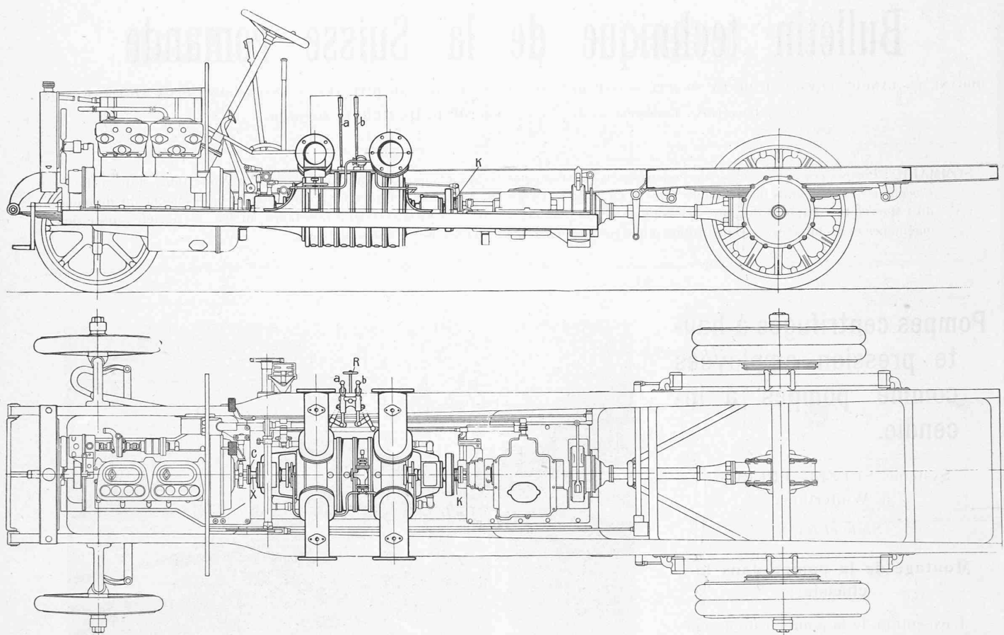
Fig. 13. — Pompe à incendie automobile « Adler ».
