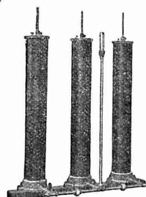
Résistance liquide.
