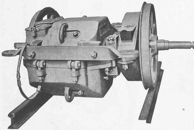
Fig. 6. — Moteur de traction.
