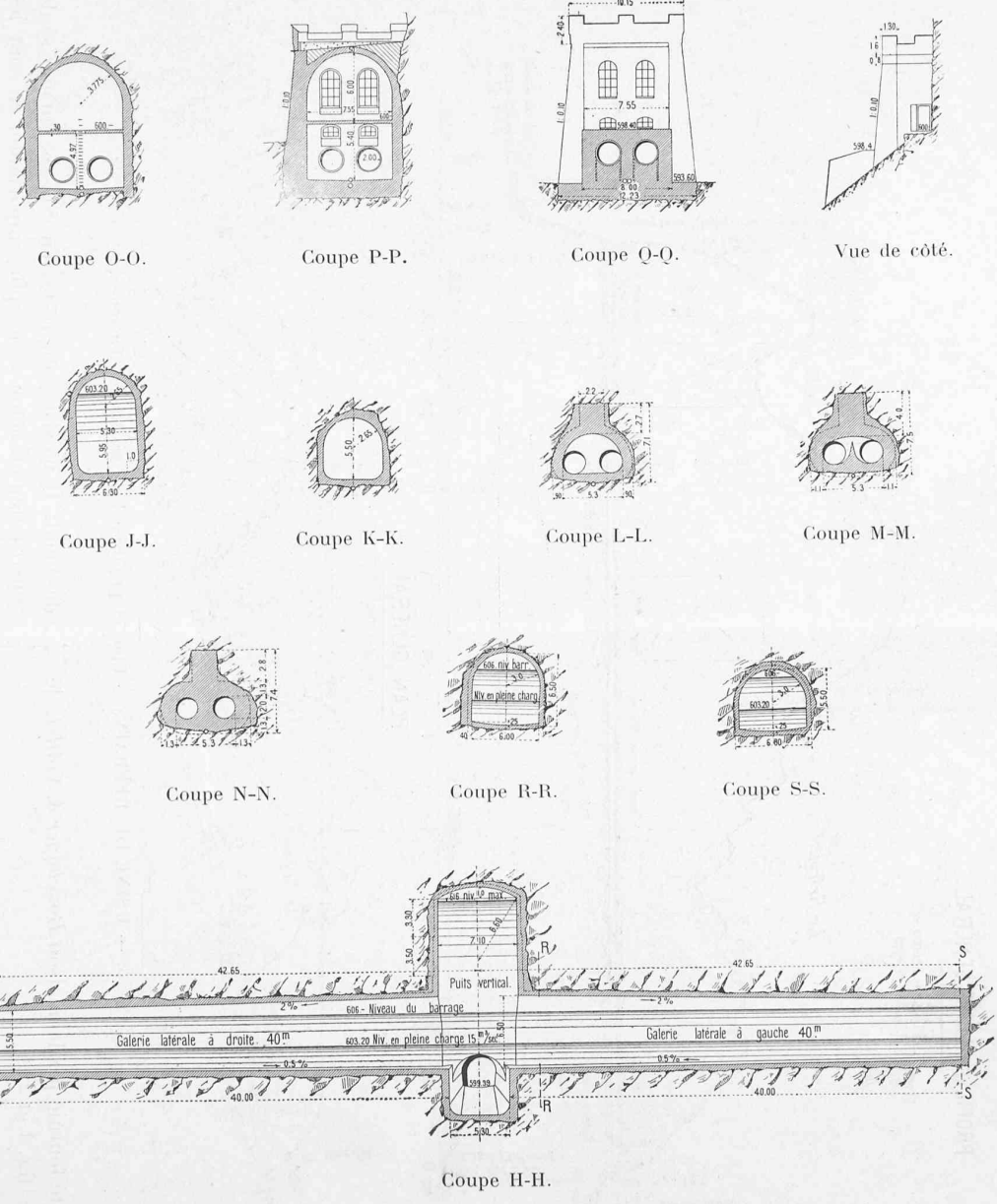
Fig. 4. — USINE DU REFRAIN. — Chambre d'eau et chambre de mise en charge. — Echelle 1 : 600.
