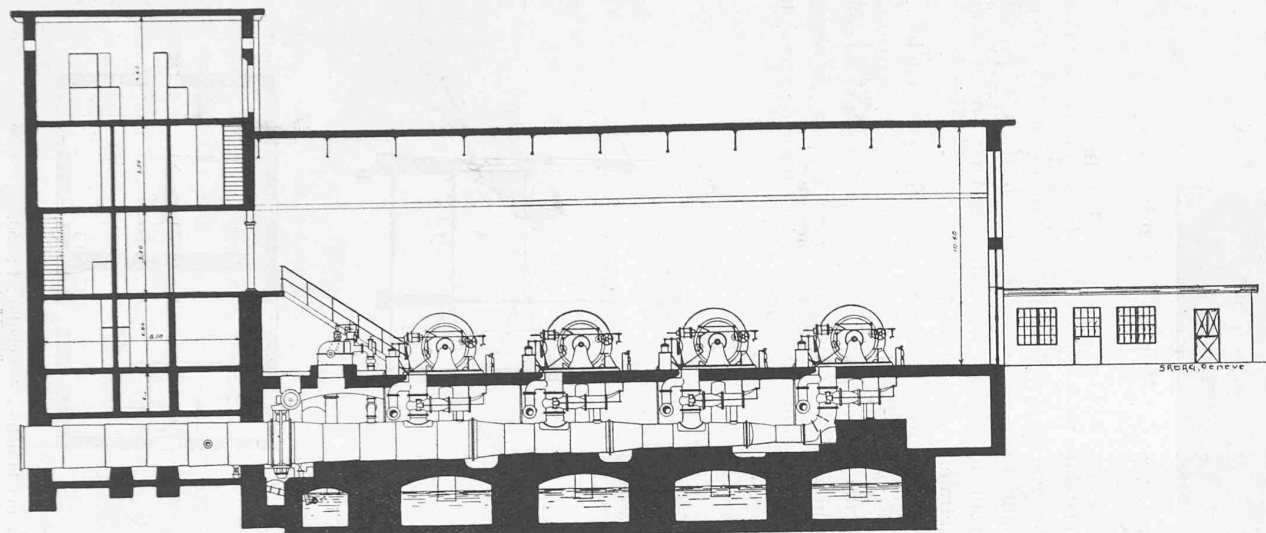
Coupe longitudinale.
