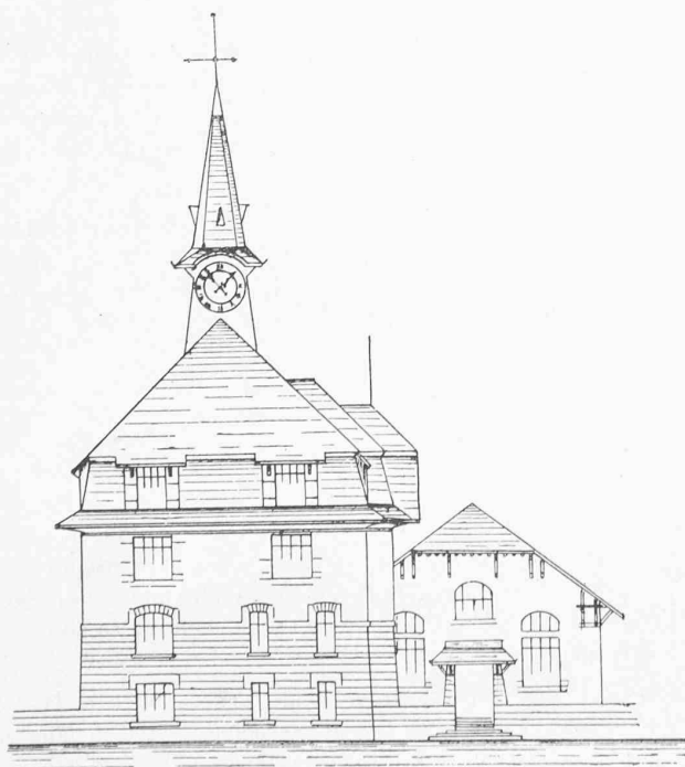
Façade latérale.
