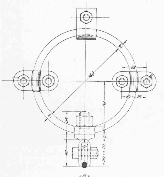
Fig. 12. — Station de Seebach. — Boucle de suspension. Prise de courant par dessous. — 1 : 3.
