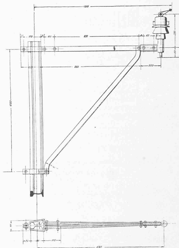
Echelle 1 : 20.
