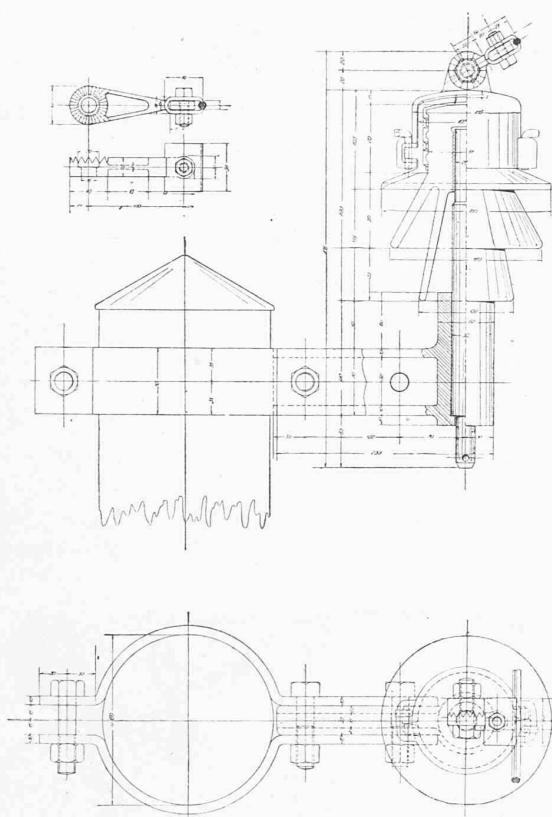
Echelle 1 : 7.
