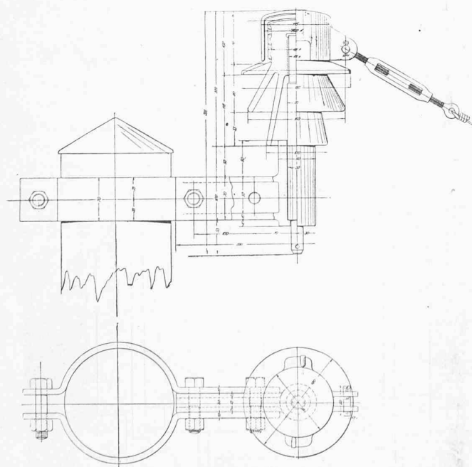
Echelle 1 : 8.
