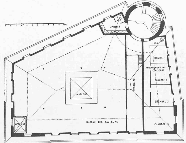
Fig. 4. — Plan du 2 me étage.
