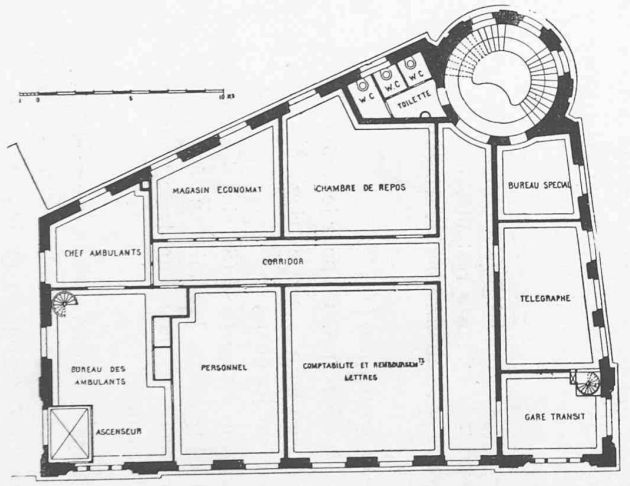
Fig. 3. — Plan du 1 er étage.
