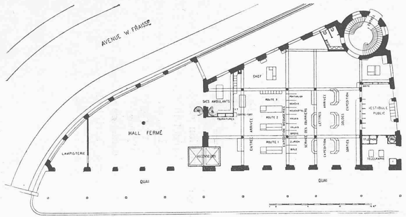
Fig. 2. — Plan du rez-de-chaussée.
