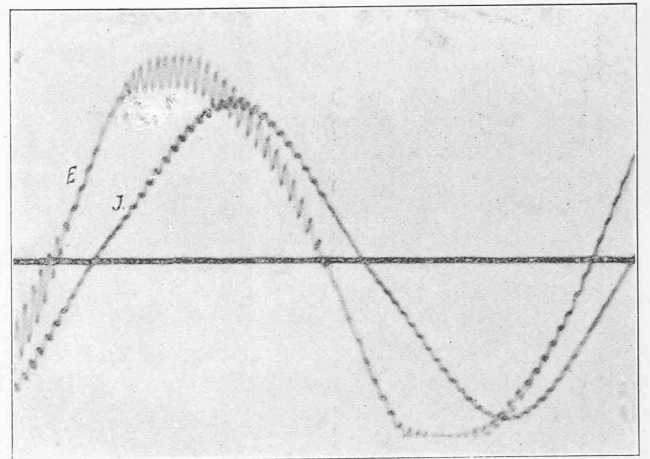
Fig. 50. — Courbes de la tension et du courant de deux générateurs en parallèle. — Locomotive N° 2 avec train de 150 tonnes, 37 kilomètres à l'heure, 64 oscillations par période. — Moteurs avec anciens induits à rainures ouvertes parallèles à l'axe.
