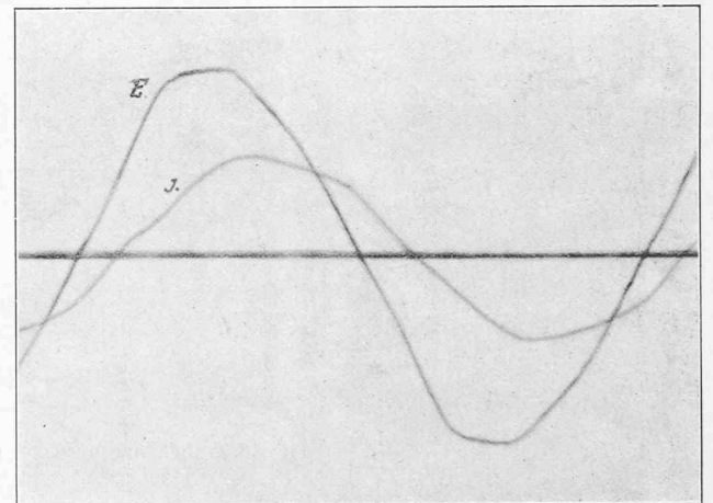
Fig. 52. — Courbes de la tension et du courant d'un générateur. — Locomotive N° 2 avec train de 50 tonnes, 43 kilomètres à l'heure. — Moteurs avec nouveaux induits à rainures fermées obliques sur l'axe.
