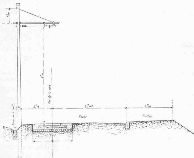
Fig. 7. — Profil-type du tronçon routier Martigny-Ville à Martigny-Bourg.
