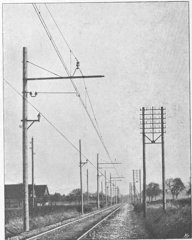
Fig. 21. — Ligne à archet latéral et ligne à suspension caténaire conduites parallèlement sur une distance de 400 m., à la sortie de la station de Regensdorf.
