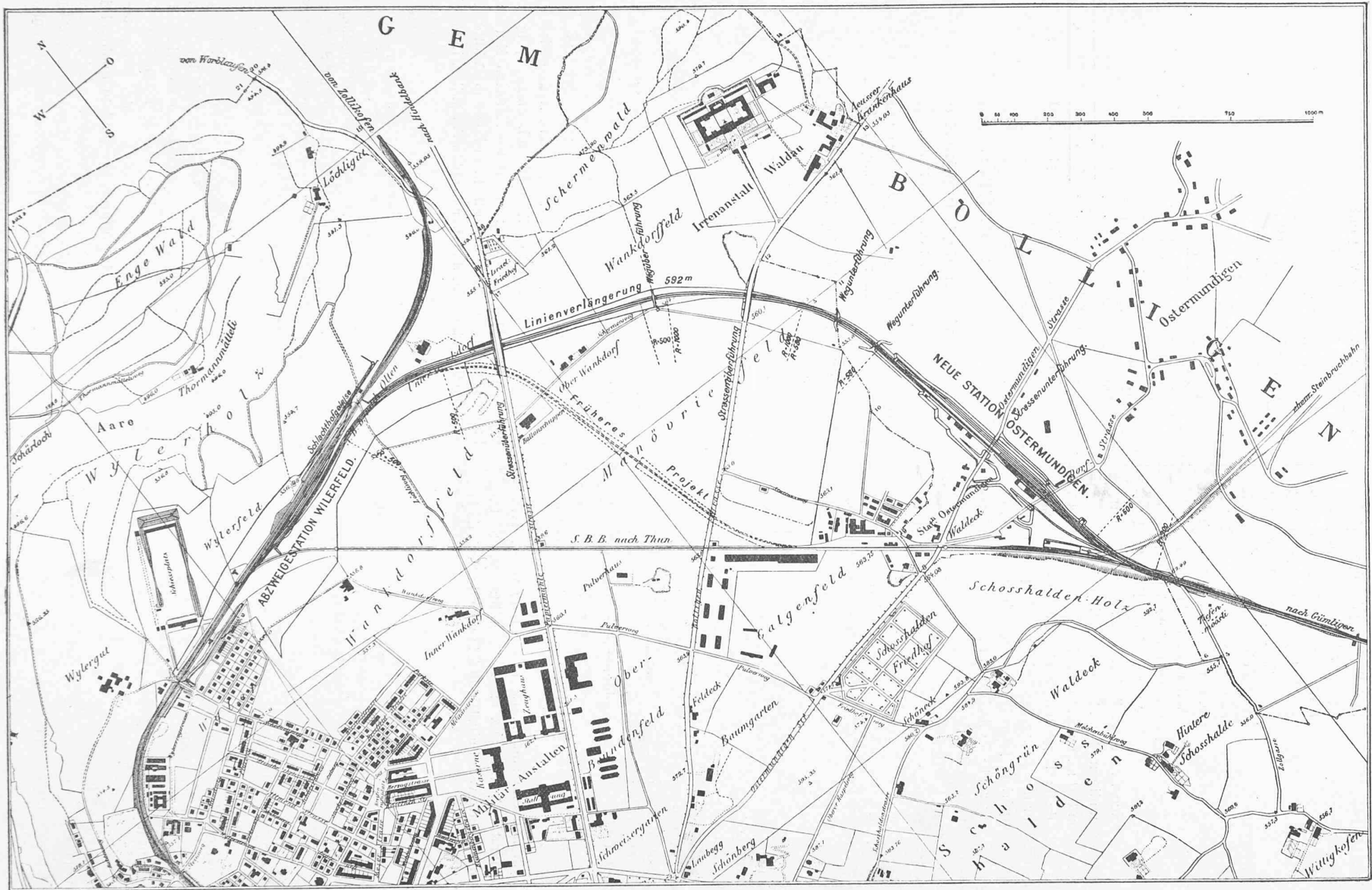
Déviation de la ligne des C.F.F. au Wilerfeld, près de Berne.
