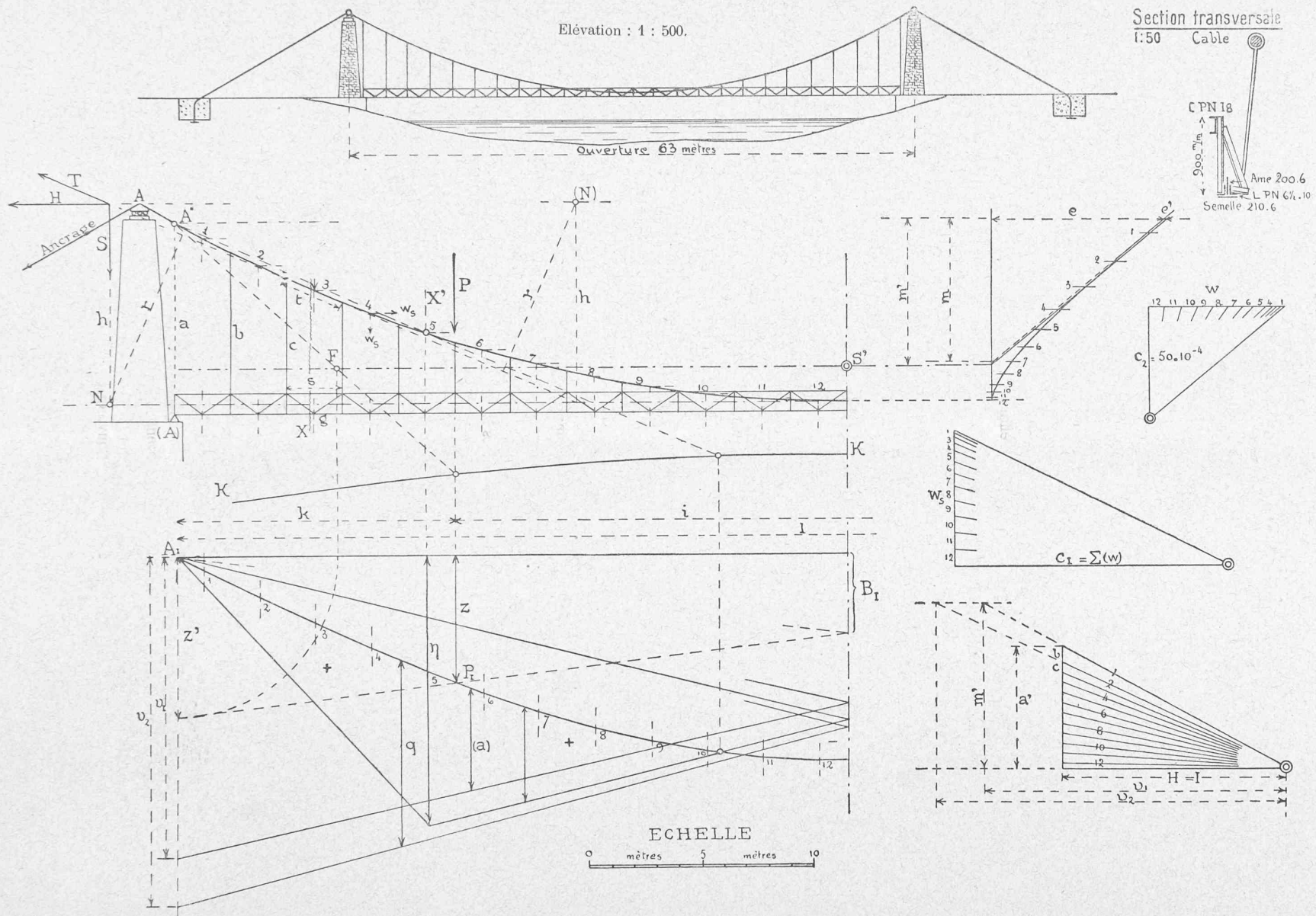
PONT SUSPENDU SUR L'ARGE, A LANGENEUGEN
