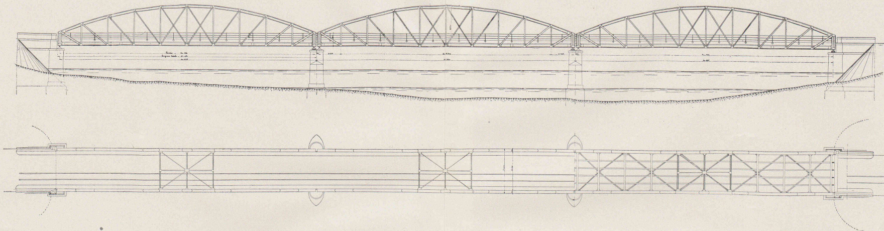
Fig. 1 et 2. — Elevation générale. — Plan.
