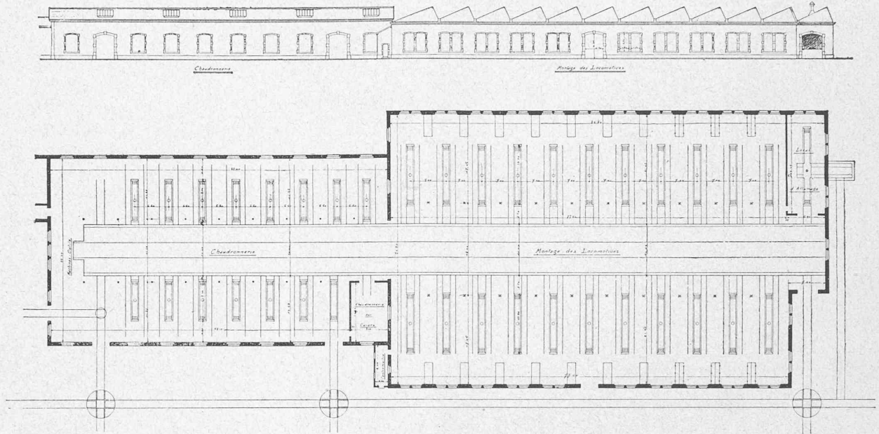
Fig. 15. — Chaudronnerie et montage des locomotives.
