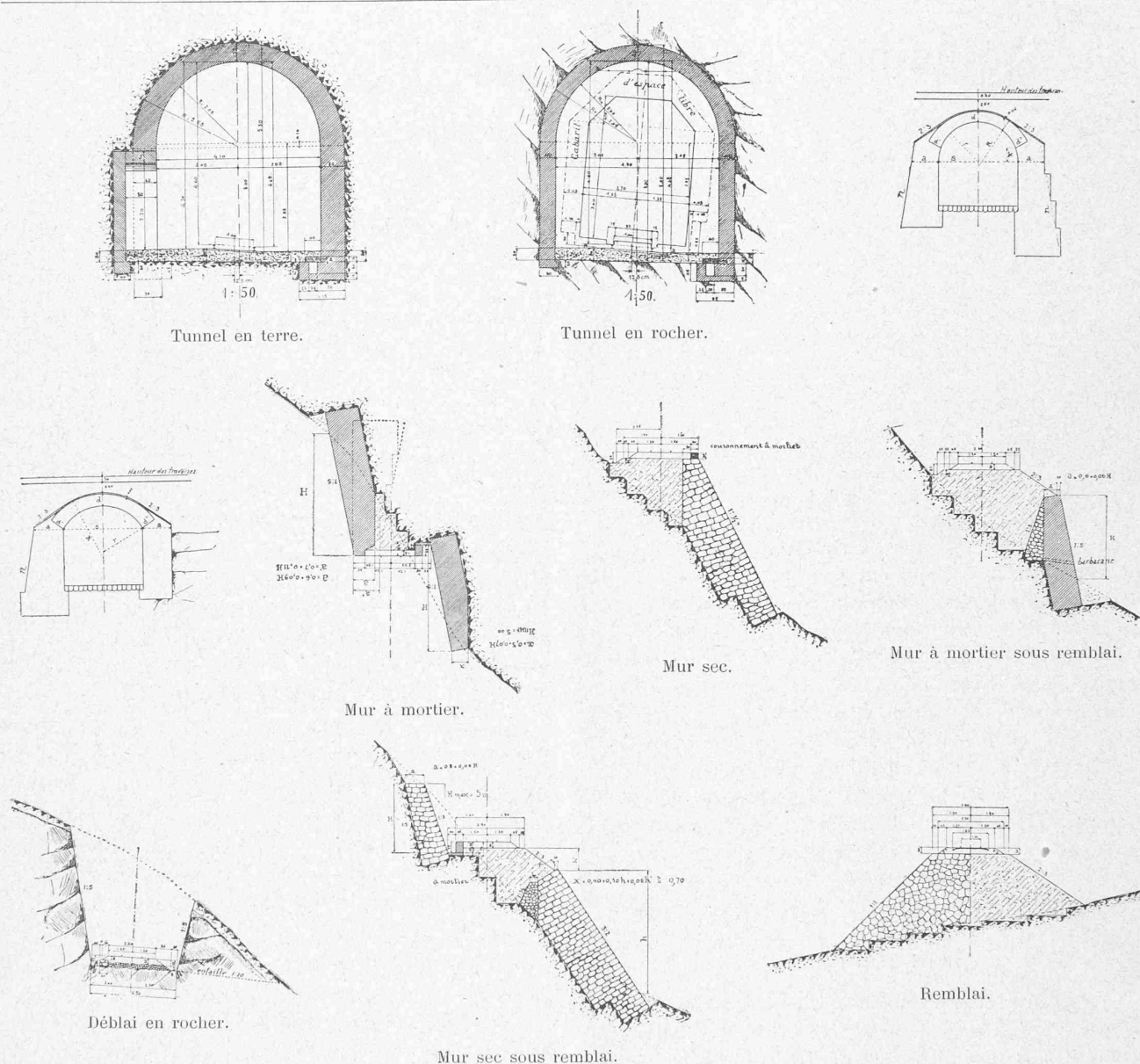
Fig. 3. — Profils-types.
