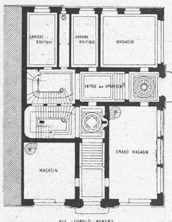
Plan du rez-de-chaussée.
