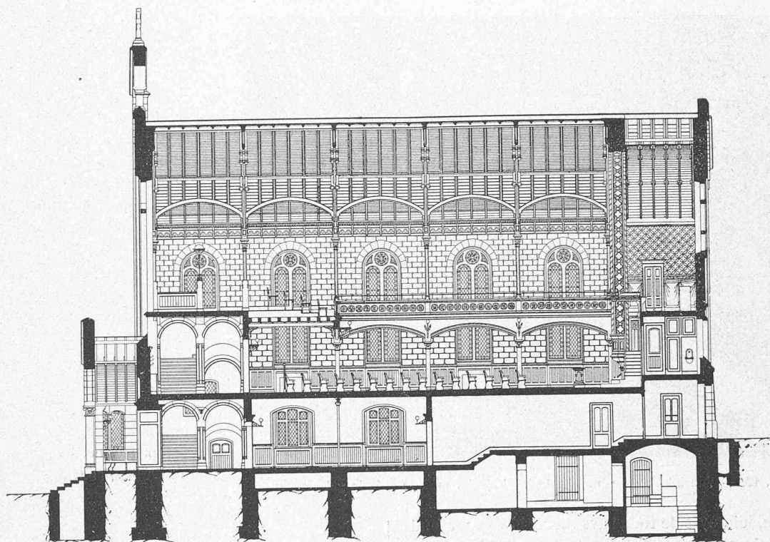
Fig. 9. — Coupe longitudinale.
