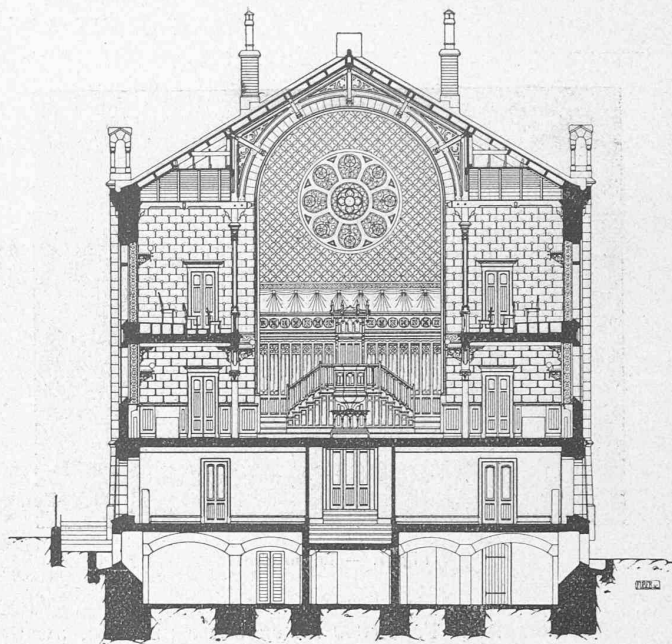
Fig. 6. — Coupe transversale.
