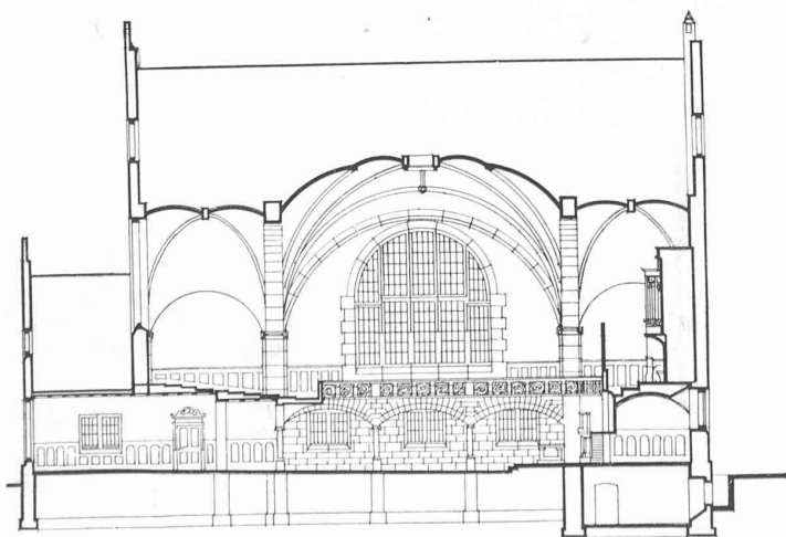
COUPE LONGITUDINALE (1 : 400)
