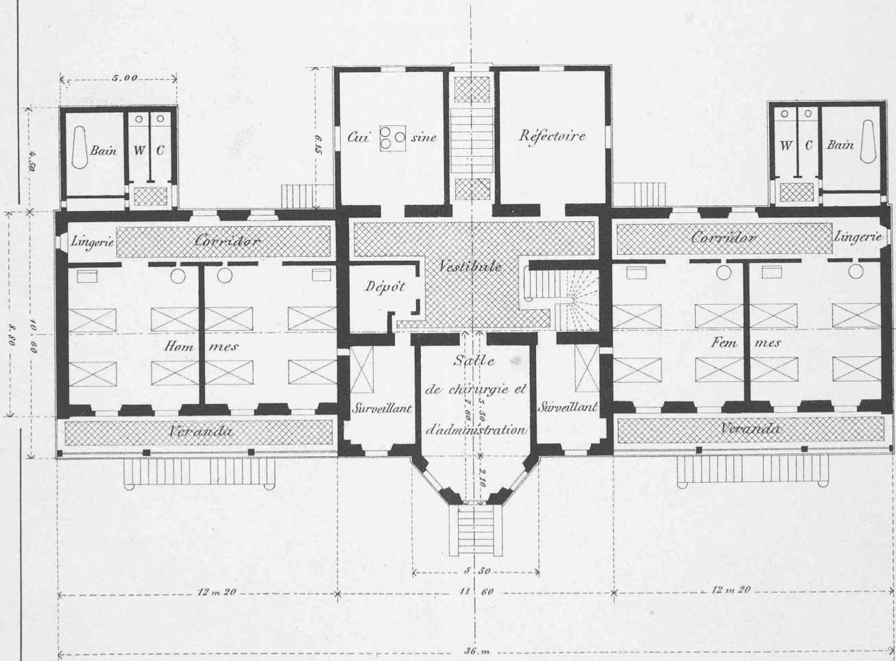
Façade sud
