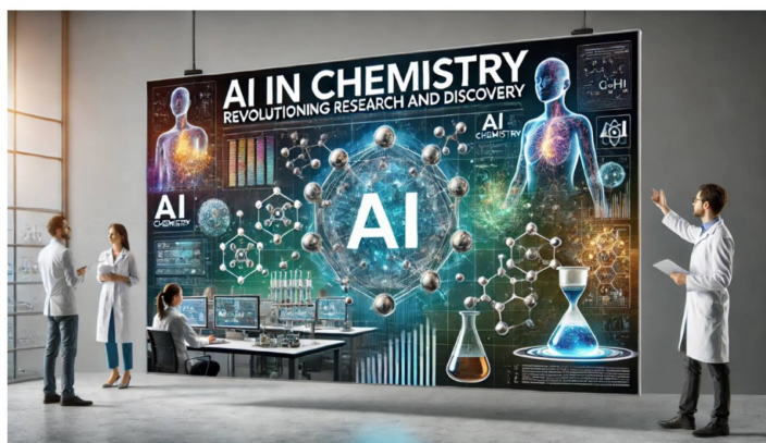
L'Intelligence artificielle au service de la chimie organique.
