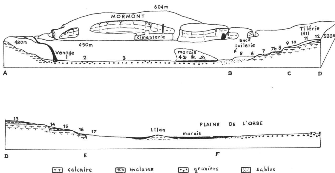
Fig. 2. — Coupe géologique de la tranchée.
