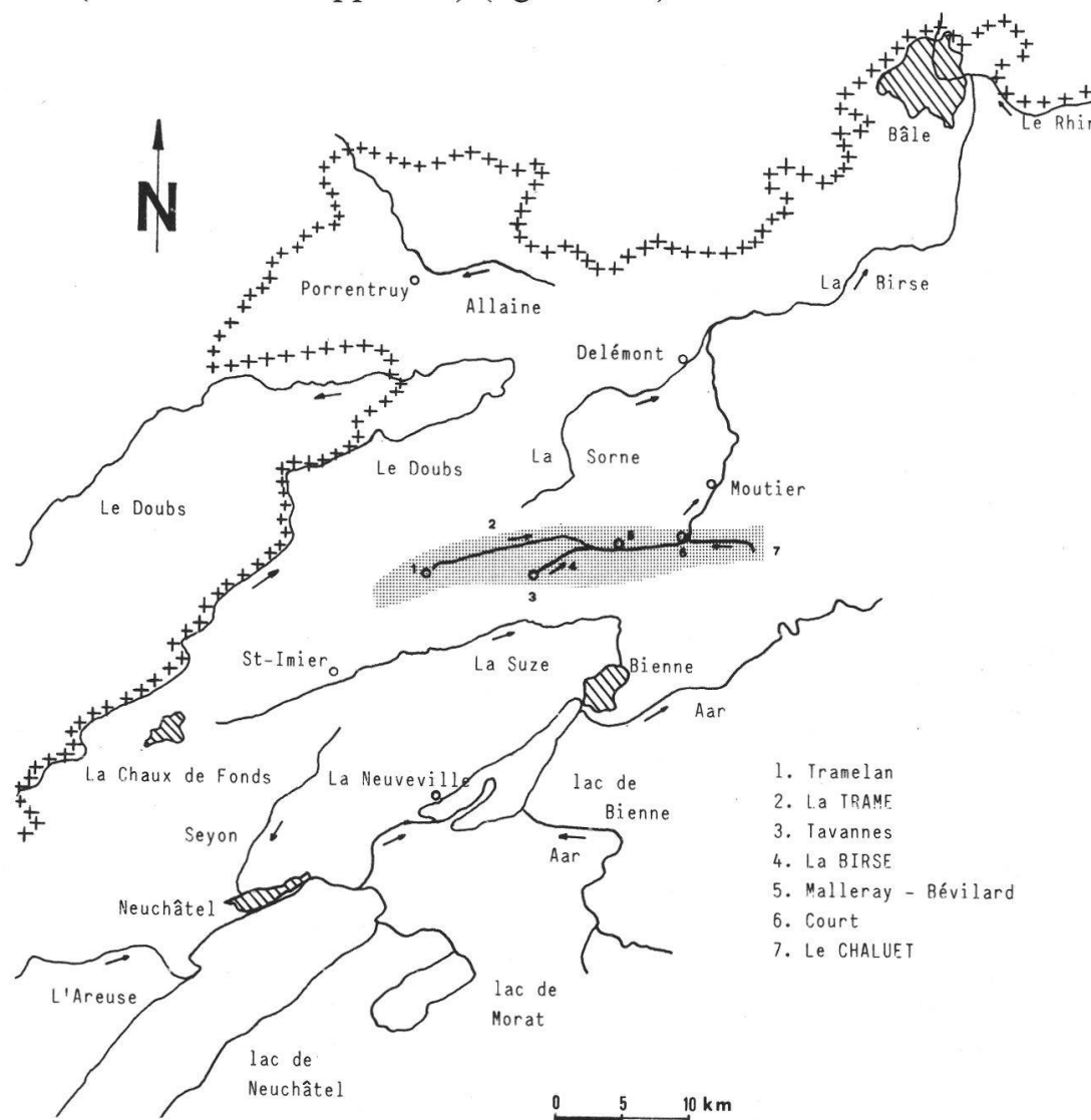
Fig. 1. Situation géographique de la Vallée de Tavannes (Jura plissé). Périmètre de l'étude. Limites du bassin — versant.
