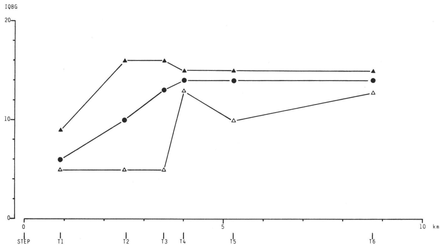
Fig. 8. Graphique des IQBG. Trame (T1 – T6). Période V.81. – IV.82.
