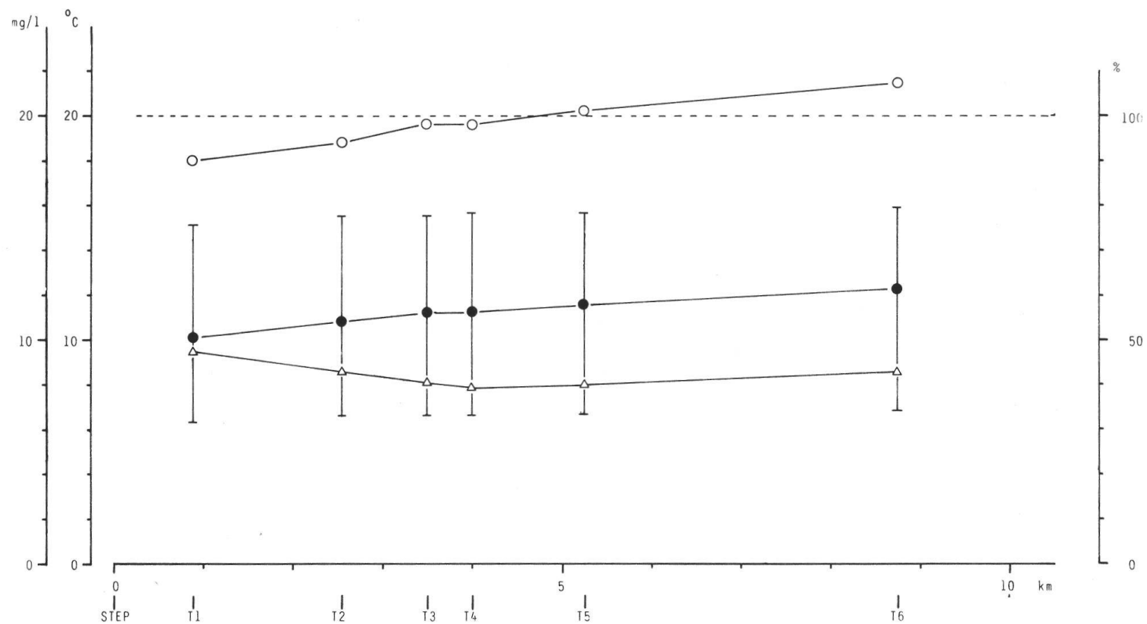
Fig. 4. Profil chimique de la Trame (T1 - T6). Période V.81 - IV.82.
