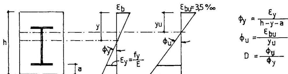
Fig1 Variation des déformations
