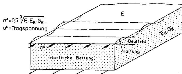
Ebene Deckbleche
