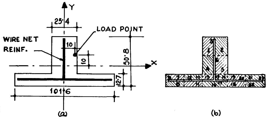
FIG. 3. ELEMENT IDEALISATION.
