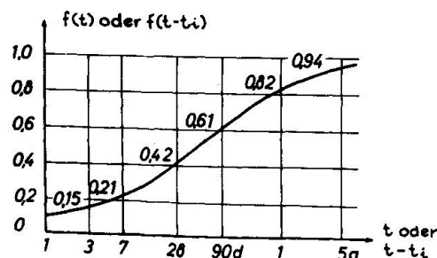
Fig. 2 Zeitlicher Verlauf der Kriech- und Schwindverformung
