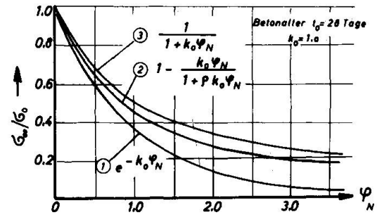
Fig. 6a \frac{\sigma_0}{\epsilon_0} bei zeitunabhängigen Zwängungen
