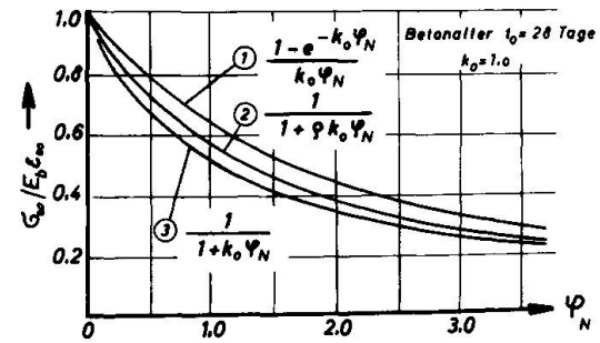
Fig. 6b \frac{\sigma_0}{\epsilon_0} bei zeitabhängigen Zwängungen, die affin zum Kriechen erfolgen
