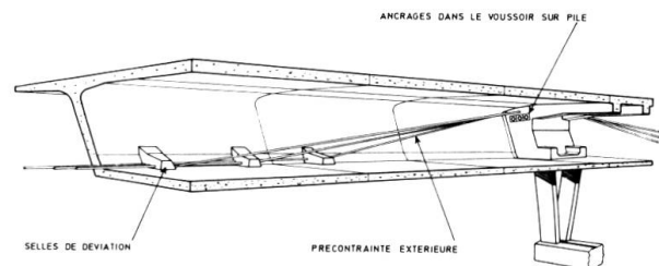
Fig. 26 - Long Key Bridge Schéma de câblage
