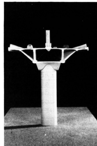
Fig. 31 - Viaduc de l'Arrêt Darré Coupe transversale - Projet SECOA
