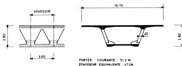
Fig. 18 - Viaduc de Sylans et des Glacières (projet SECOA) Maquette et voussoir type
