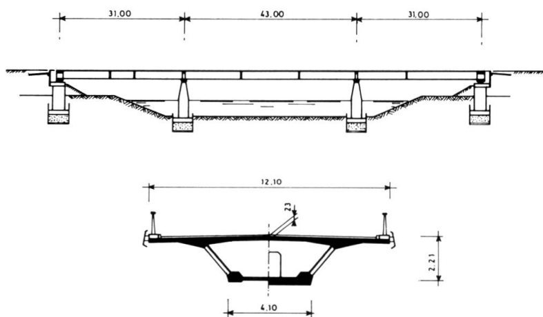
Fig. 7 - Pont de Cognac - Coupes longitudinale & transversale
