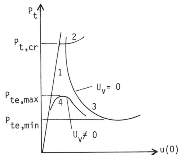
Fig. 8 Courbes d'équilibre
