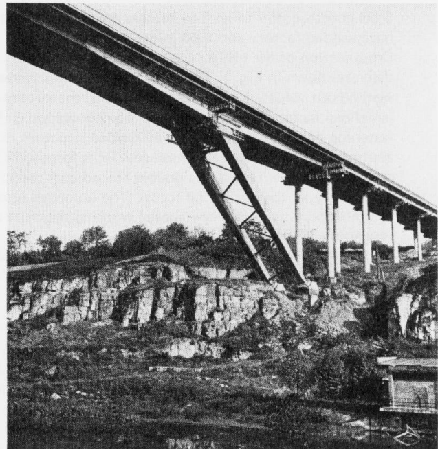
Fig. 7 Une partie de la travée centrale avec des béquilles
