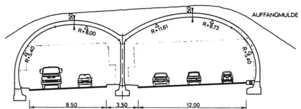
REGELQUERSCHNITT TUNNEL MIT KRIECHSPUR
