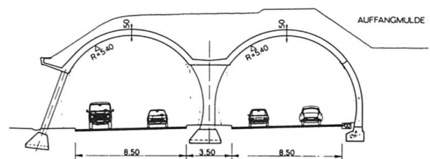
REGELQUERSCHNITT OFFENE GALERIE
