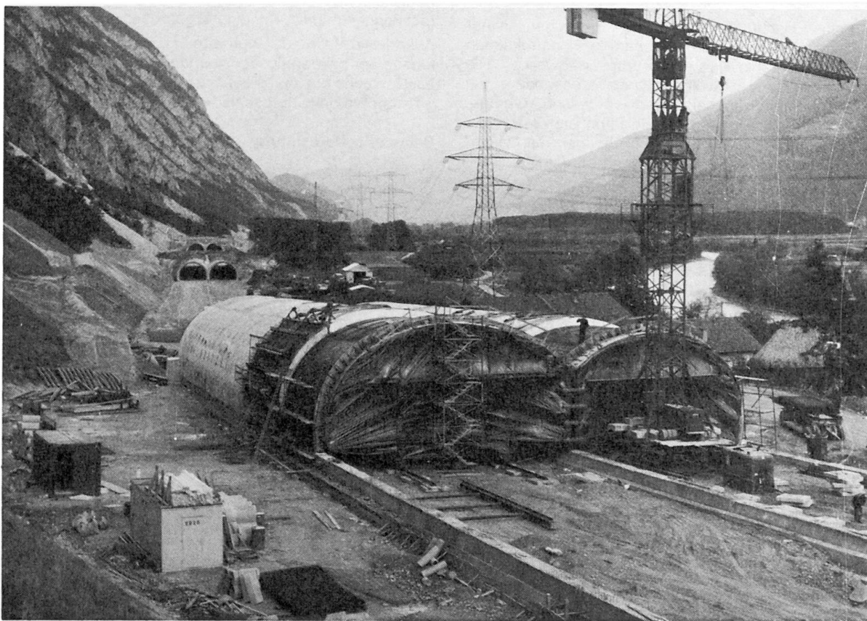
Bild 3 Tunnel mit Kriechspur
