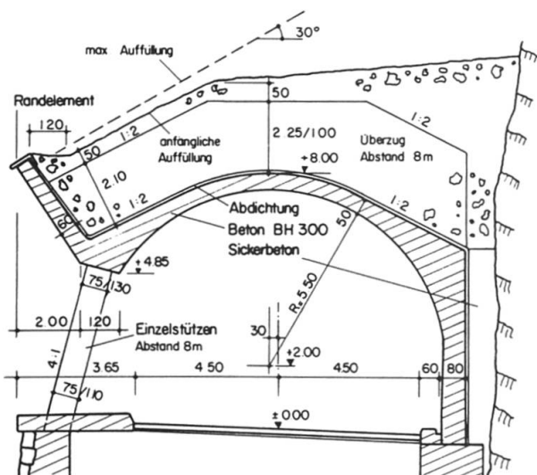
Bild 1 Galeriequerschnitt
