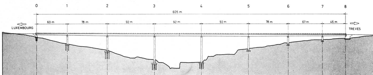
Fig. 2 Coupe longitudinale
