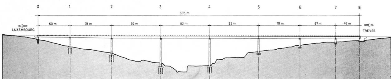
Fig. 2 Coupe longitudinale
