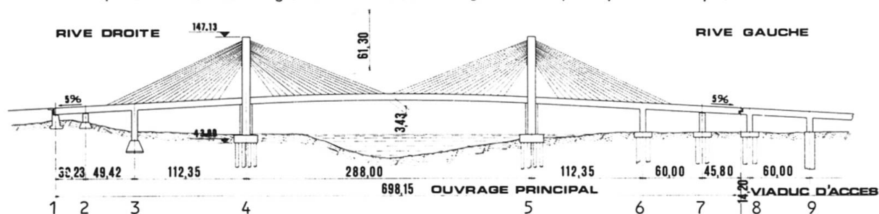
Fig. 1 Coupe longitudinale
