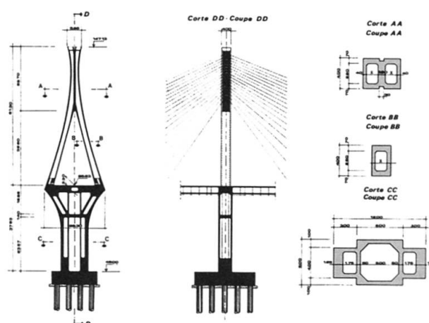
Fig. 2 Piles principales — Coupes
