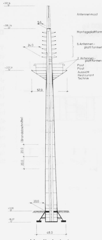
Vertikalschnitt
