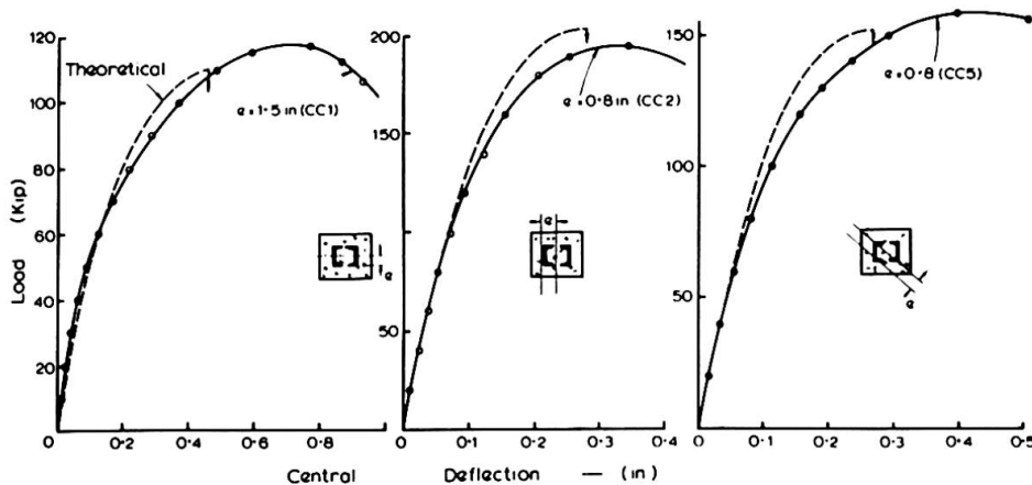
FIG. 11 BATTEN COLUMNS
