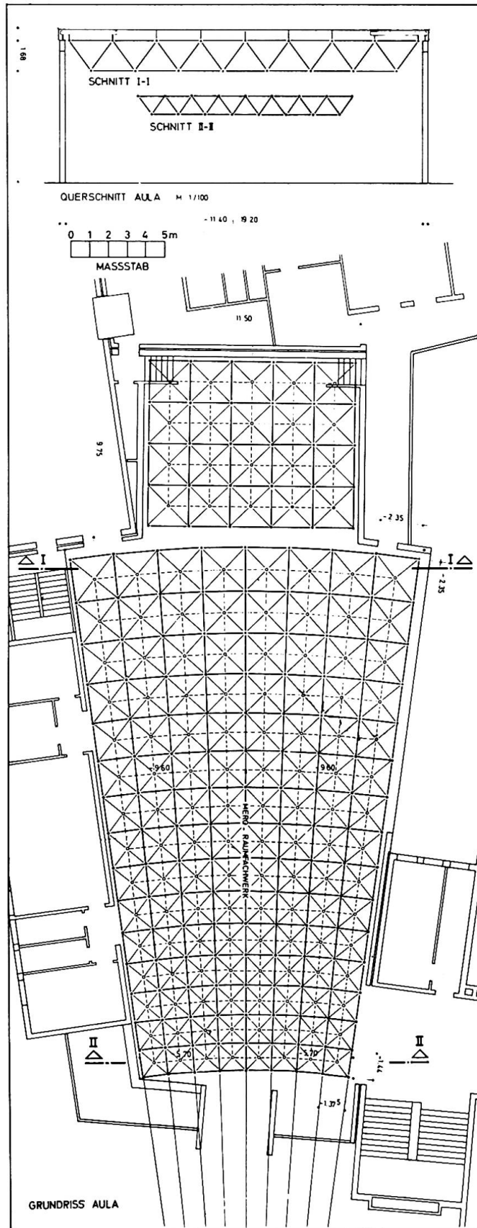
Bild 7: Raumbachwerk für eine Aula mit trapez-förmigem Gesamt-Grundriss und Trapez-Raster (gebildet durch eine Schar parallel laufender Geraden, die sich auf einem Fluchtpunkt ausserhalb des Gebäude-Grundrisses schneiden). Die Bauhöhe der einzelnen Elementarkörper ändert sich im Verhältnis der Trapez-Seiten. Dr. 923
