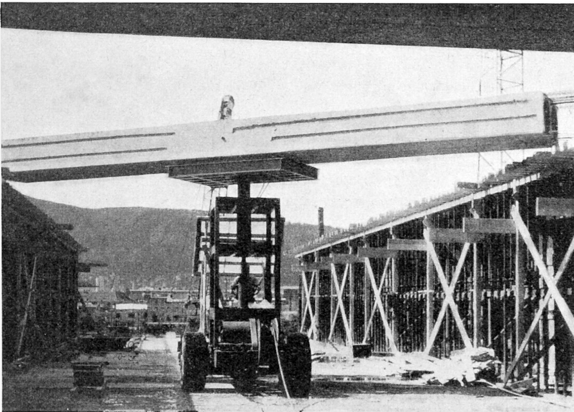
Abb. 4 - Montage von 18 t schweren Hohlplatten mit speziell angefertigtem Versetzgerät auf einer Baustelle in Herdern bei Zürich. Ingenieur: R. Henauer und J. Lee, Zürich. Unternehmer: Locher & Cie AG, Zürich.
