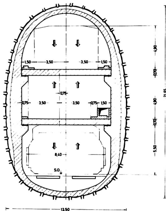
Bild 3: Tunnelquerschnitt (Vorschlag E des Ing.-Büro Berger)
