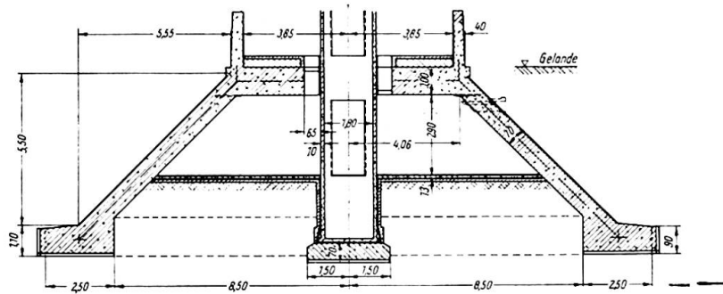
Fig. 16 Fundament des Fernmeldeturmes Hannover nur mit Kegelstumpfschale
