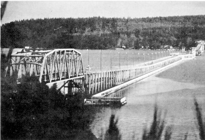
Abb. 1 zeigt als Beispiel für eine "schwimmende Balken-Brücke" die Brücke über den Hood-Kanal in den USA.
