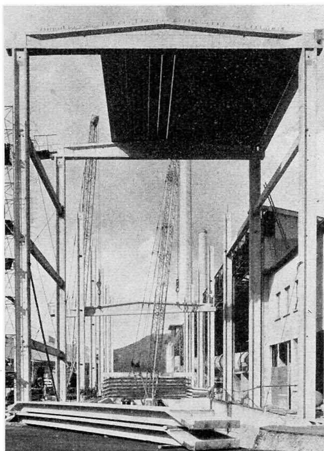
Abb. 6 - 20 m hohe Industriehalle aus vofabrizierten BBR-I-Profilen und Balkenplatten in Wildeg. Ingenieur: E. Schubiger, Zürich. Vofabrizierte Elemente: Stahlton AG, Zürich.
