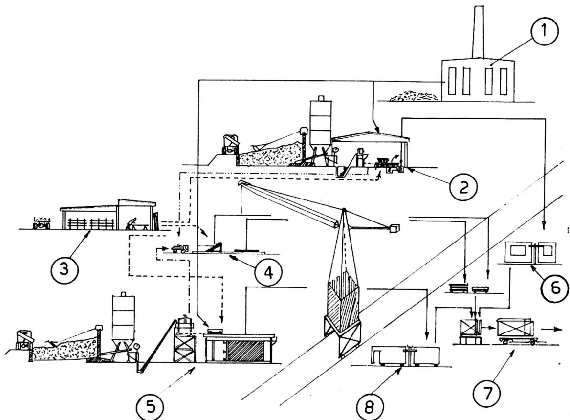
Bild 13 - Produktionsablaufschemata für ein Betonwerk, das auf die komplette Herstellung von Gebäuden spezialisiert ist (mehrere Technologien nach Abschnitt 3.1.1 bis 3.1.3): 1, Dampferzeugung (Heizhaus) - 2, Aussenwandelemente (Kippformfertigung) - 3, Schweisserwerkstatt - 4, Ergänzungselemente (Einzelformfertigung) - 5, Innenwandelemente Deckenelemente (Batterieformfertigung) - 6, Lager - 7, Palettenabsetzbühne oder andere Fahrzeuge - 8, Lager.
