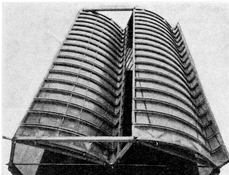
Abb. 8 - Modellversuch eines aus Segmenten zusammengesetzten Schalensdaches für eine inzwischen ausgeführte Überbauung in Wangen bei Olten. Ingenieur: H. Hossdorf, Basel. Vorfabrikation Element AG, Veltheim AG.
