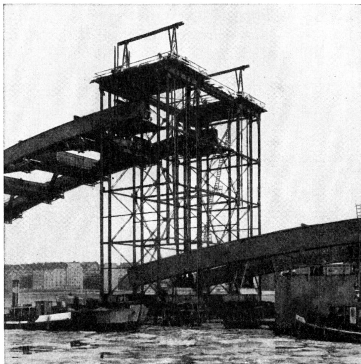
Fig. 8. Pont de l'Ouest. Tour provisoire pour le levage des arcs.
