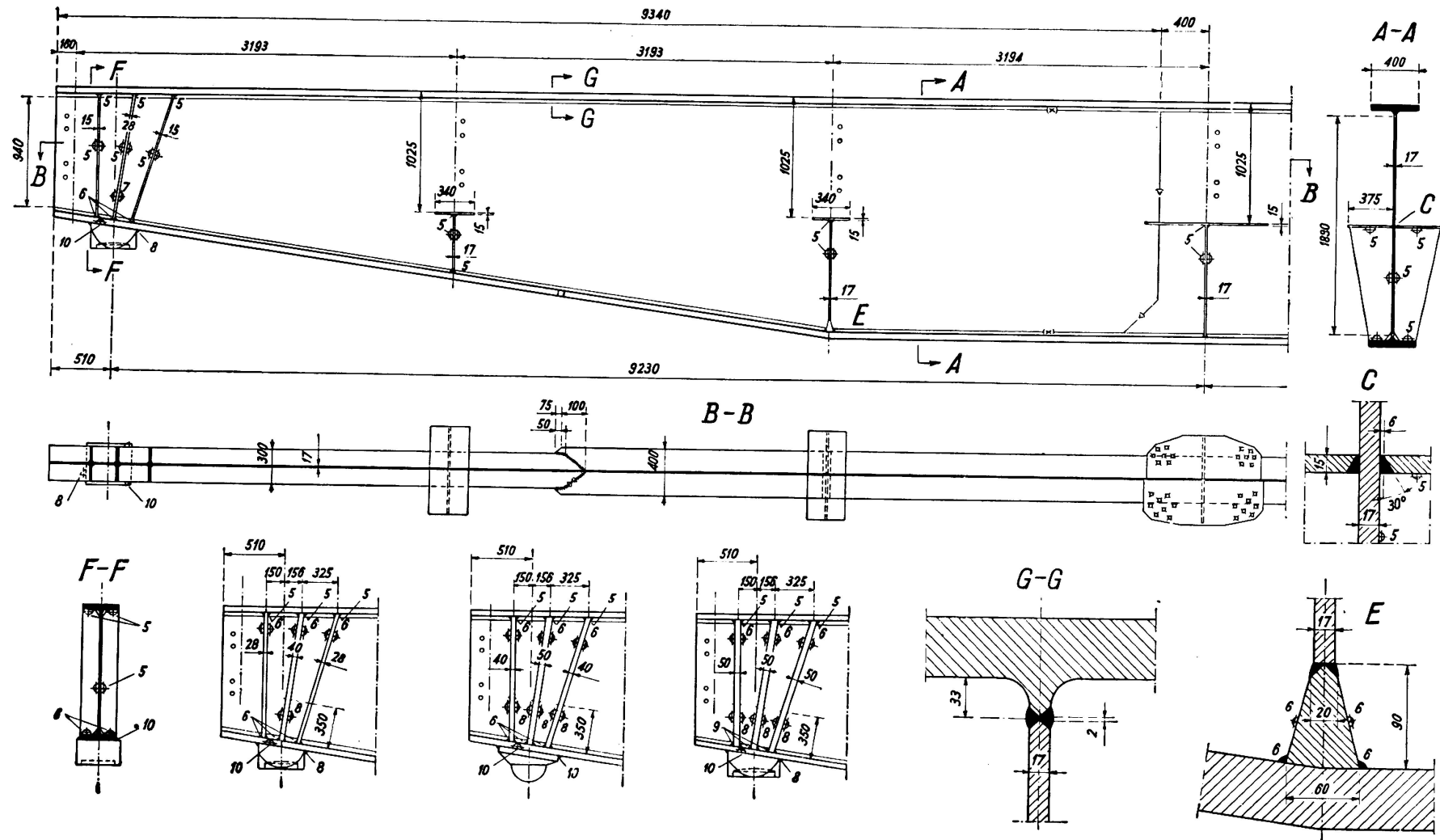
Fig. 11. Pont de Pälund. Entretoises.
