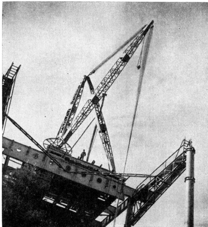
Fig. 9. Pont de l'Ouest. Montage des travées de rive.
