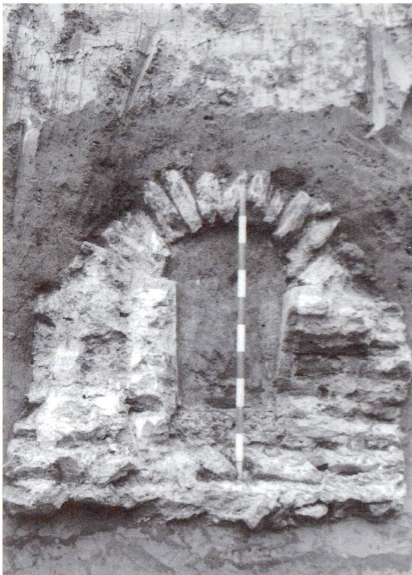
Fig. 27a. Photo de l'aqueduc de Coppet au point C.16.
