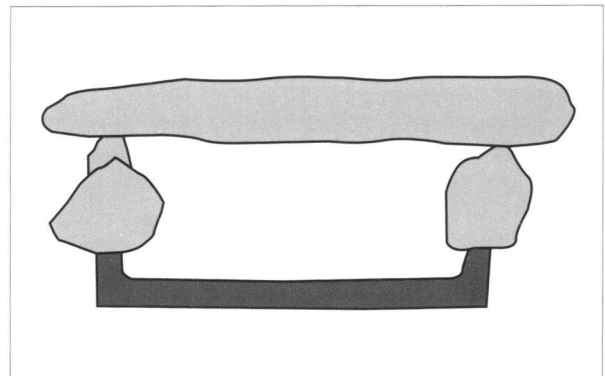
Fig. 10. Coupe de la conduite secondaire de l'aqueduc de Bonne Fontaine au point BF.S.2. Sans échelle. (cf. fig. 7b).
