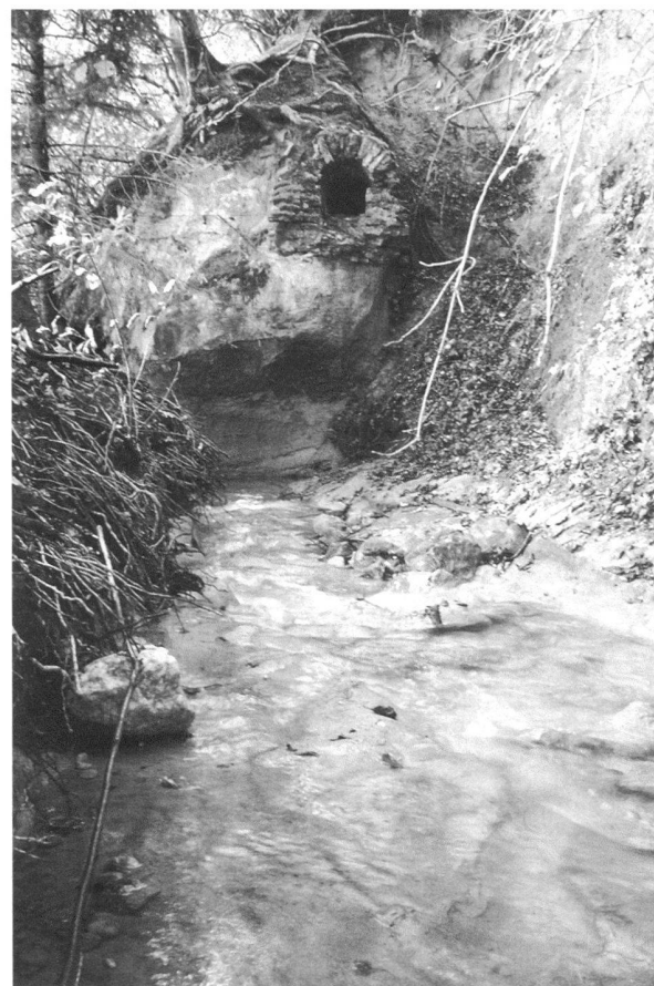
Fig. 21a. Photo de la conduite de Coppet sortant de la roche au point C.7.
