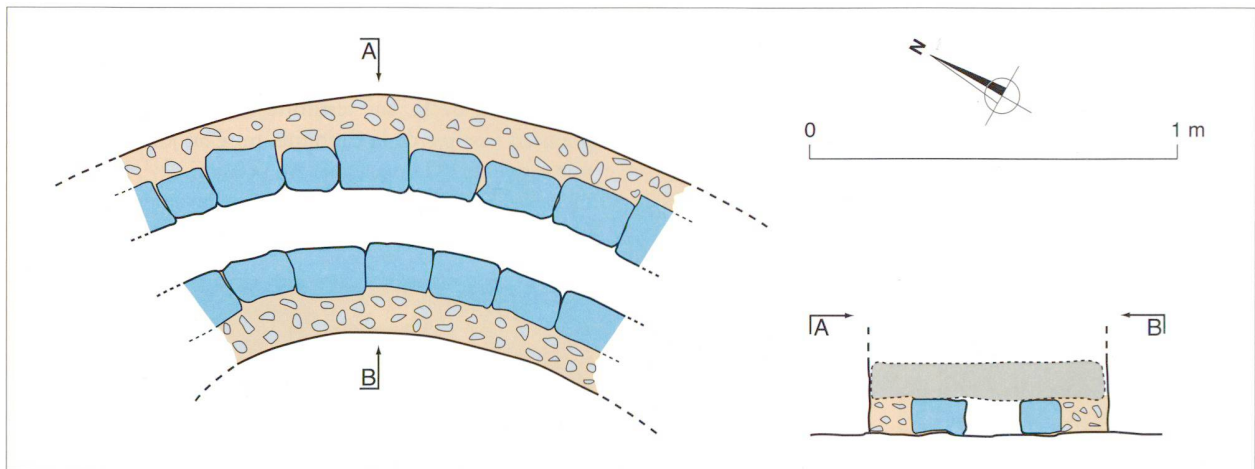
Fig. 17. Plan et coupe de la conduite secondaire de l'aqueduc de Coppet au point C.S.2. Echelle: 1:20. (cf. fig. 7b).
