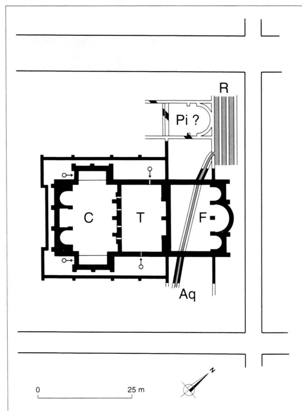
Fig. 34. Plan des thermes d'En Perruet à l'état I. Aq: aqueduc, C: caldarium, F: frigidarium, P: palestres, Pi: piscine, R: citernes, T: tepidarium. Sans échelle.
