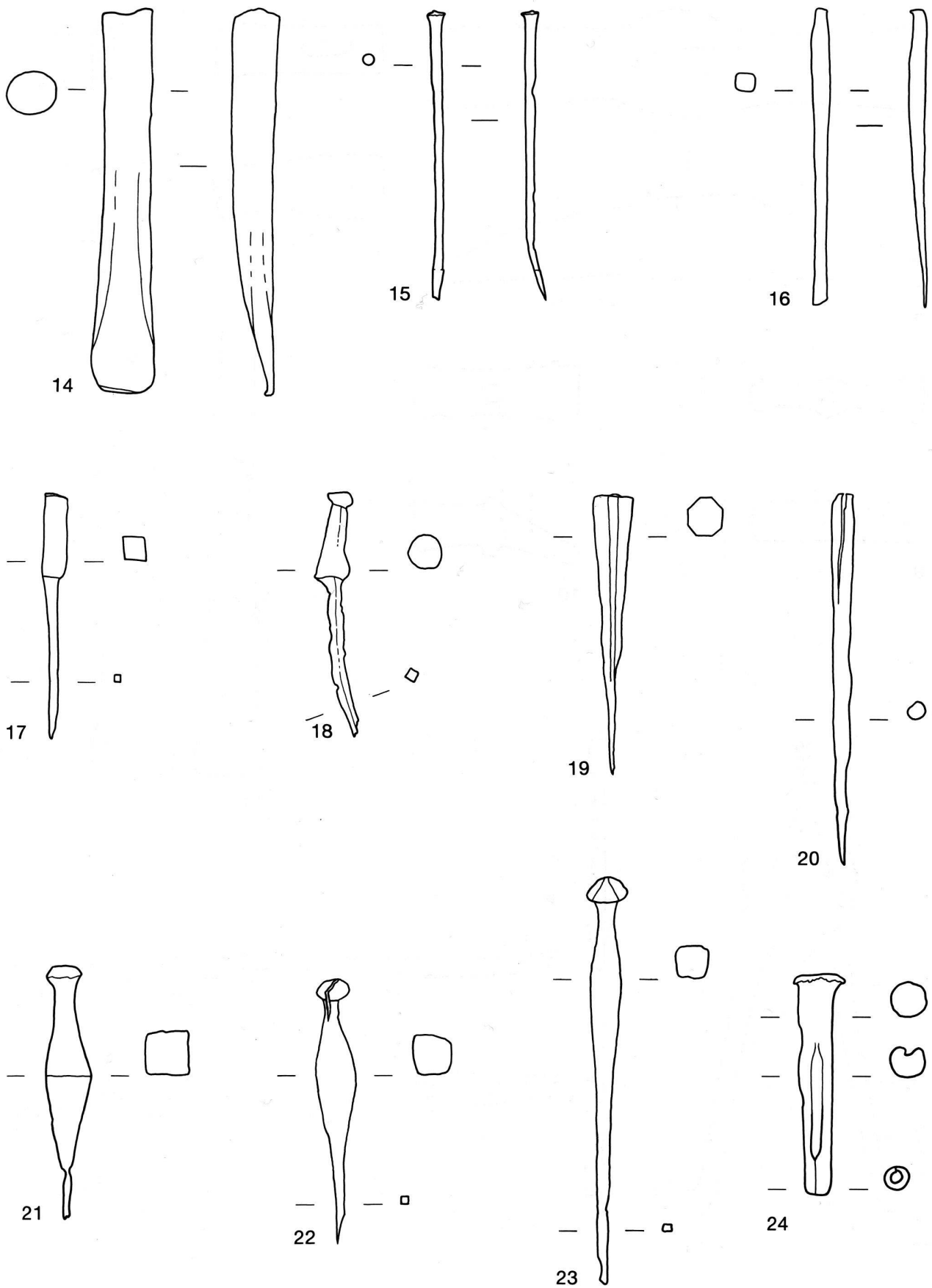
14: ciseau droit; 15-18: ciselets; 19-23: poinçons; 24: emporte-pièce Ech.: 1:2
