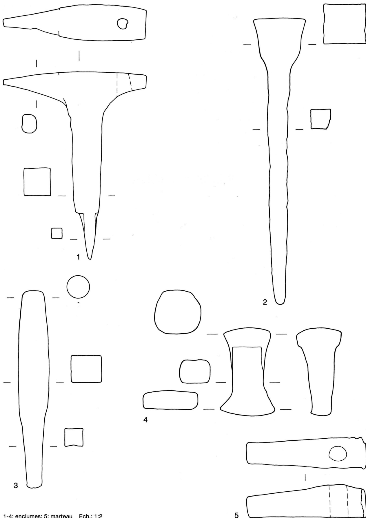
1-4: enclumes; 5: marteau Ech.: 1:2
